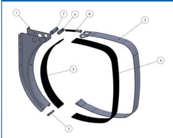
Réf. KIT Montage : 7169 0000 B
