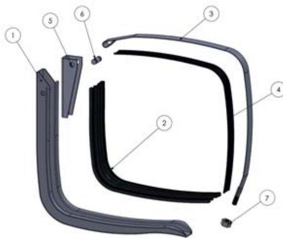
Réf. KIT Montage : 7171 0000 B
