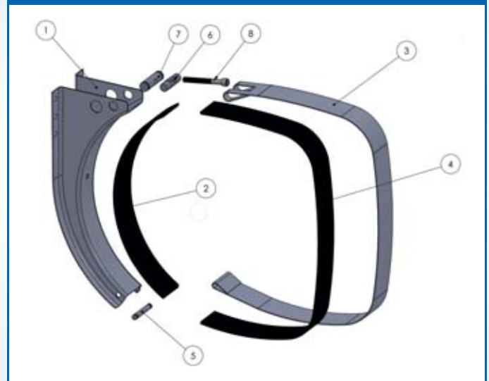
Réf. KIT Montage : 6856 0000 B
